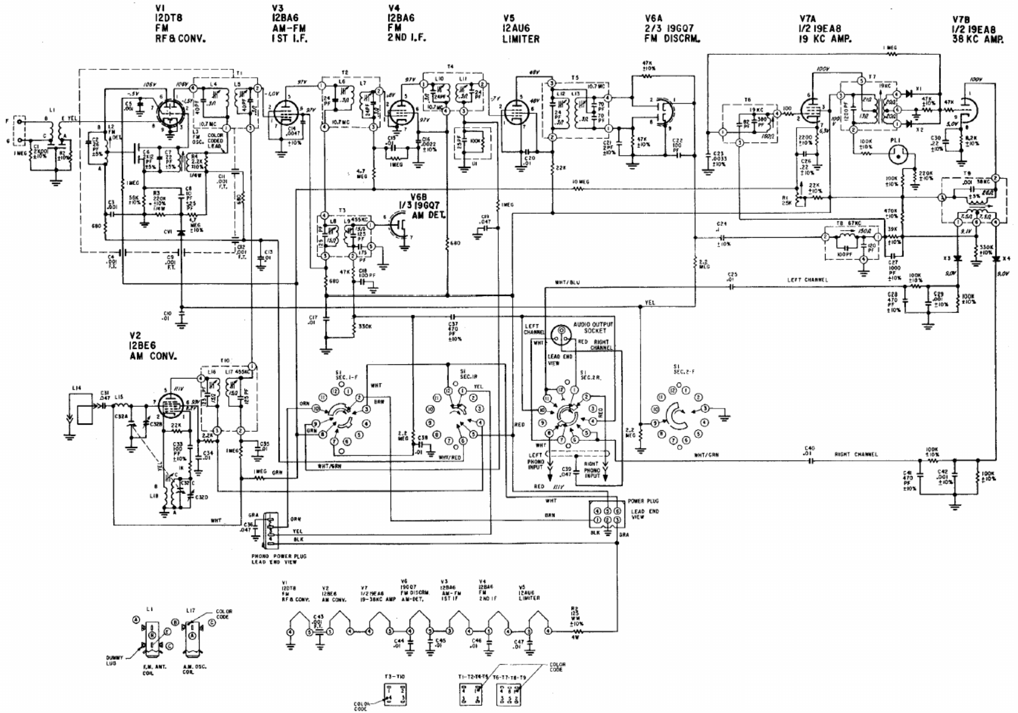
ZENITH Mod. ML2420-3, ML2601-3, ML2602-3 e ML2603-3 CON DECODER 7L01
